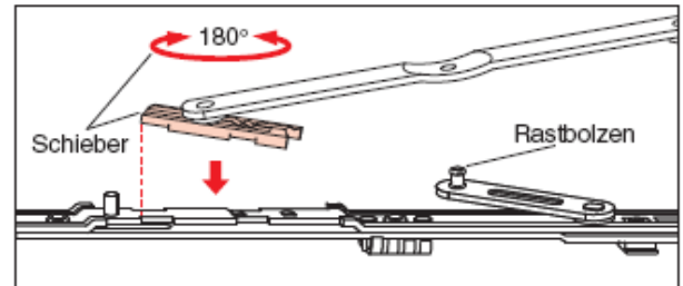
Kippweite reduziert (80 mm)
