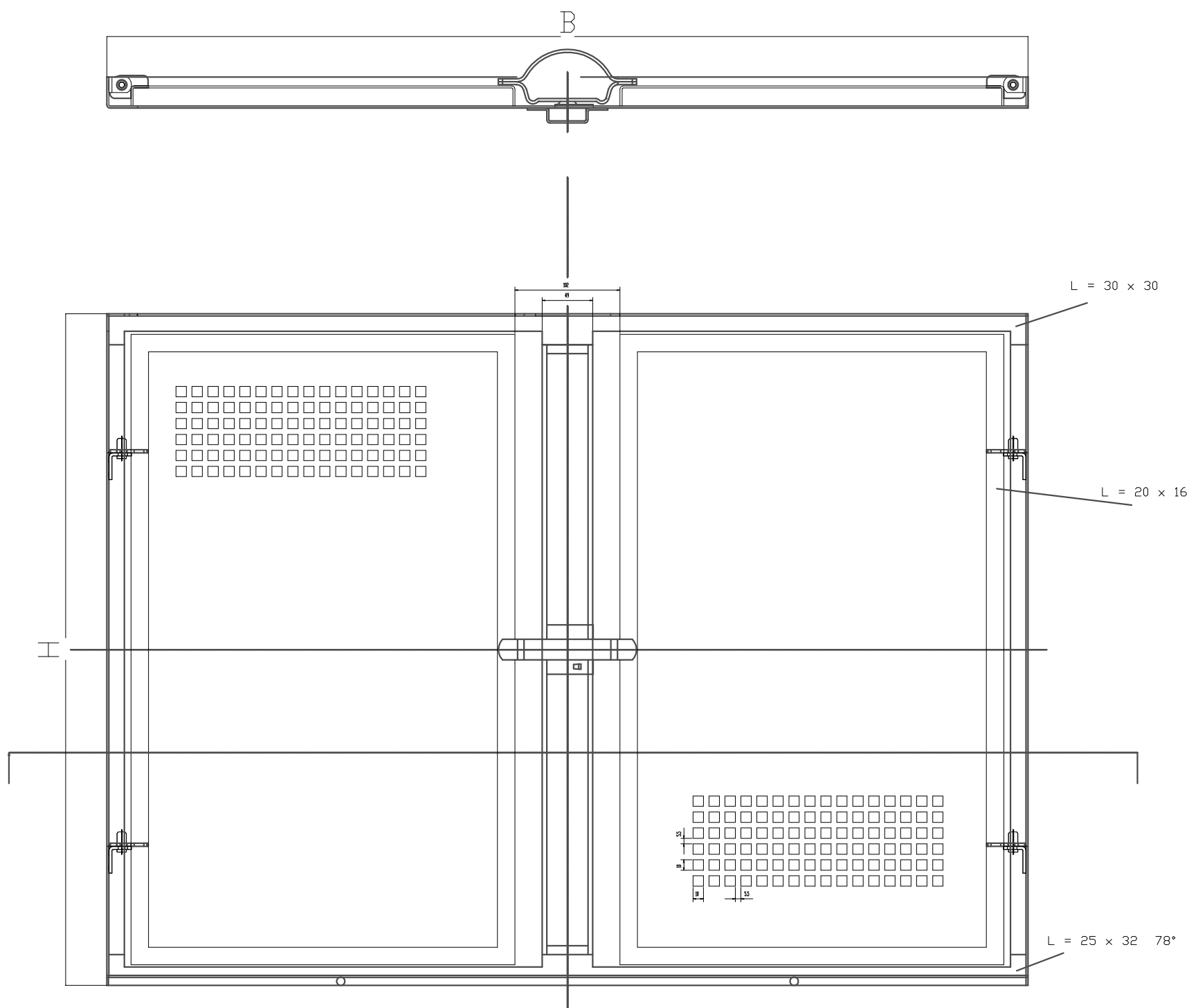
Stahlfenster
