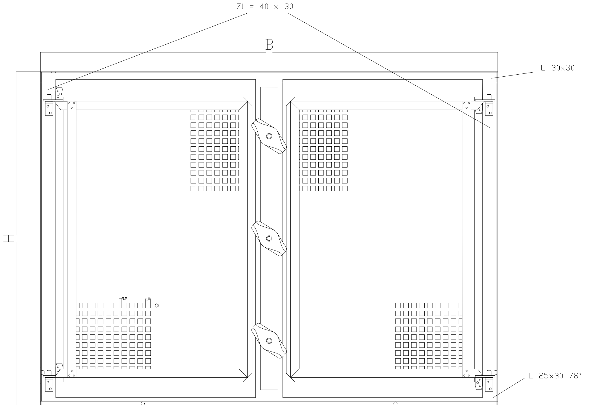
Stahlfenster
